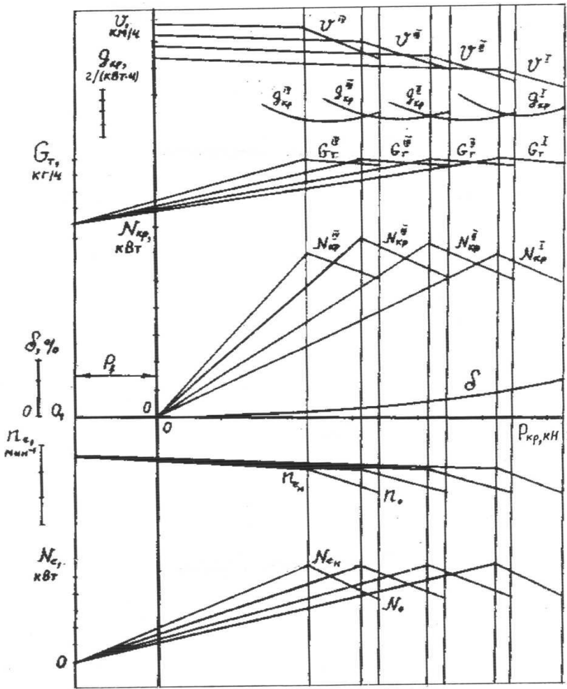
Рисунок 1.1 – Теоретическая тяговая характеристика трактора
